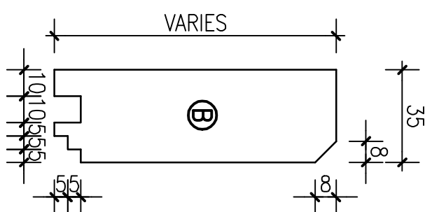
SECTION D-D
