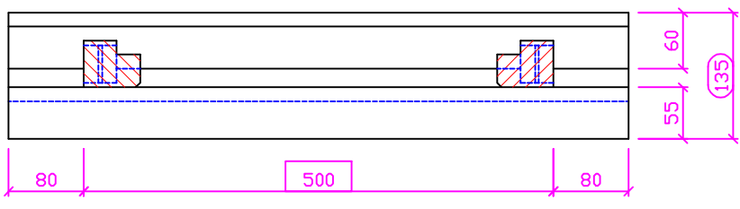
B-B
