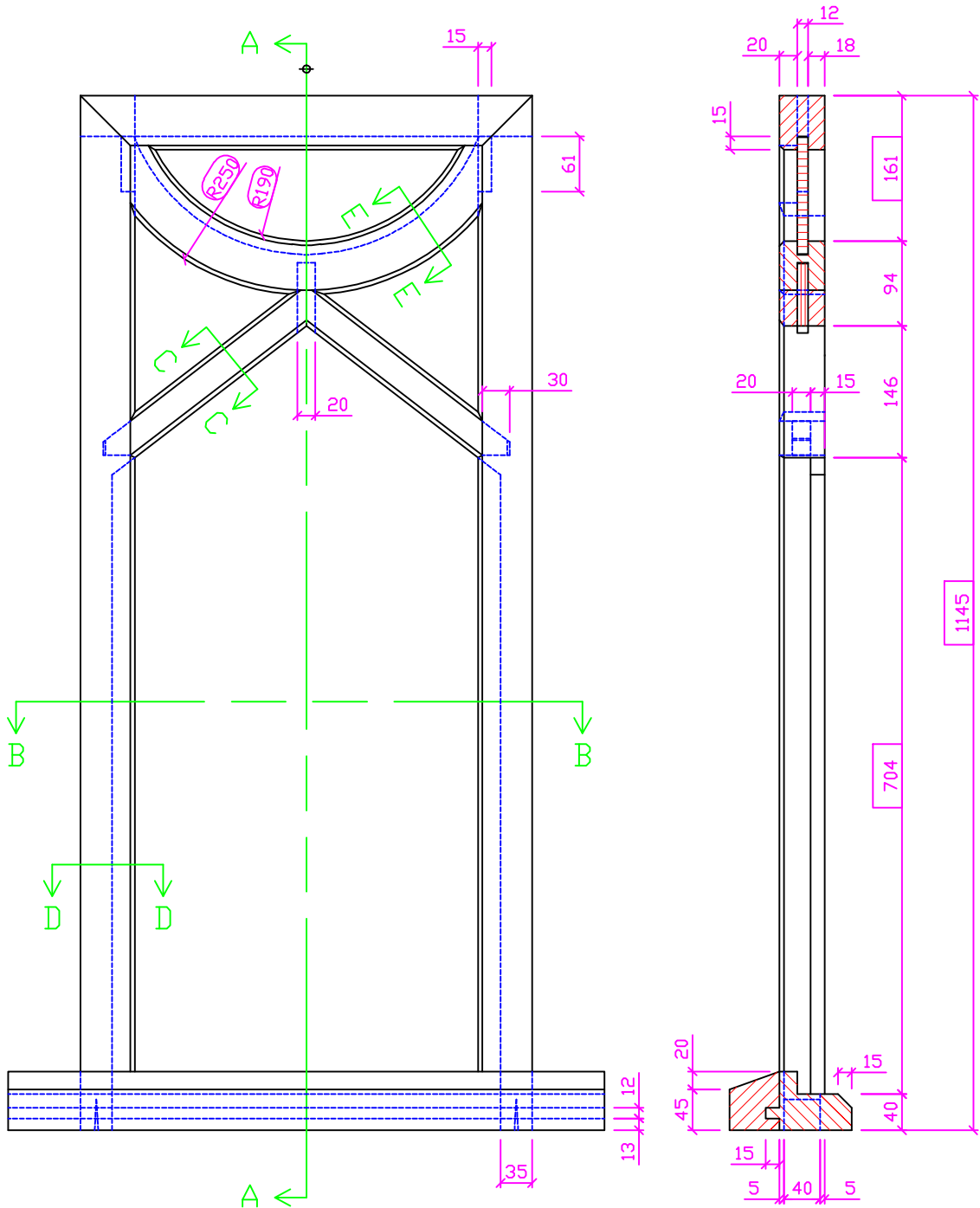
A-A
