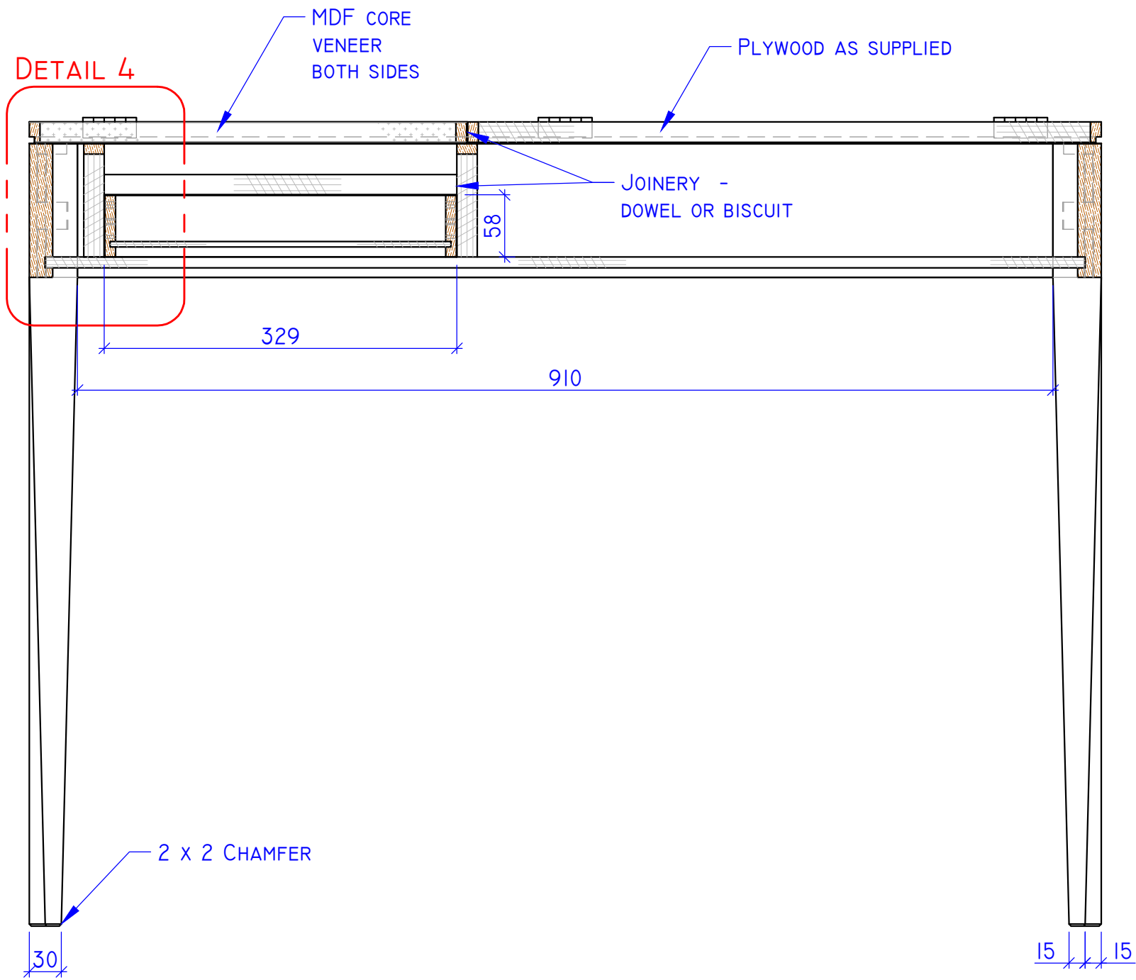
SECTION B : B SCALE 1 : 5
